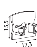
Tapa/End cap
